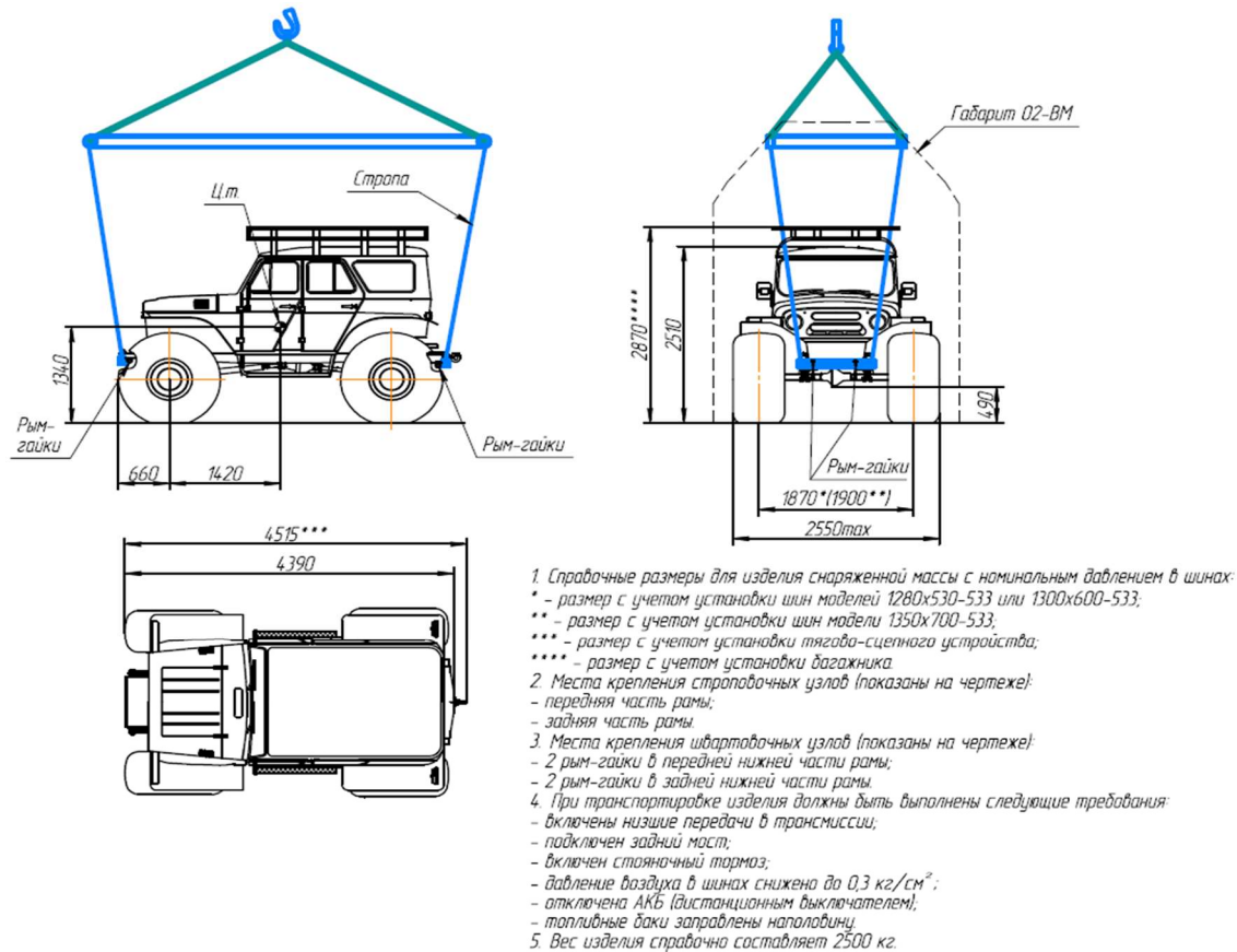
Рис. 15 Схема расположения строповочных и швартовочных узлов ВТС
