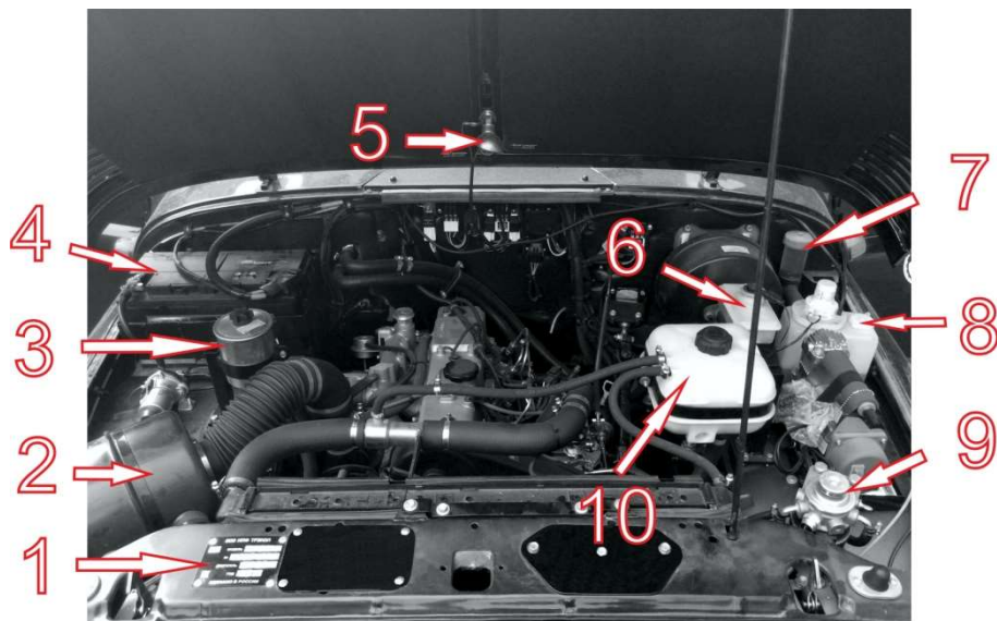
Рис. 4.1 Подкапотное пространство:
