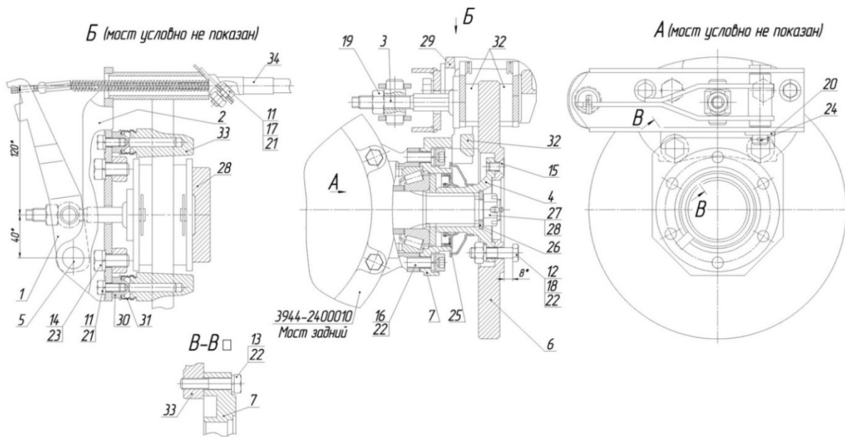
Рис. 6.6 Устройство стояночного тормоза
