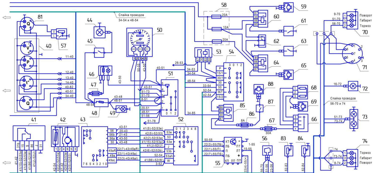
Рис. 6.7 (часть 2) Базовая электрическая схема ВТС
