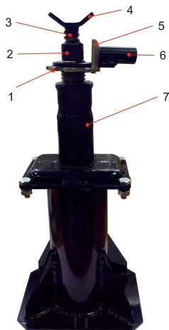
Рис. 12.1 Домкрат:
