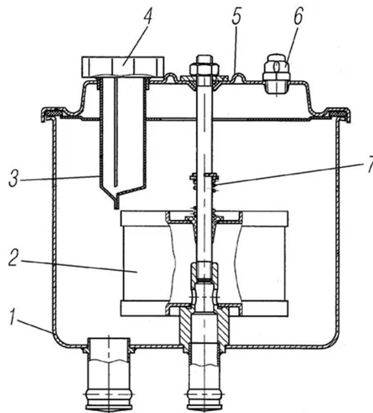
Рис. 6.5 Бачок усилителя рулевого управления: 1 – корпус; 2 – элемент фильтрующий; 3 – фильтр заливной; 4 – пробка; 5 – крышка; 6 – клапан предохранительный; 7 – пружина фильтра.
