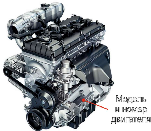
Рисунок 4.5 Модель и номер бензинового двигателя ЗМЗ-40905.10, ЗМЗ-409051.10 и ЗМЗ-409052.10
